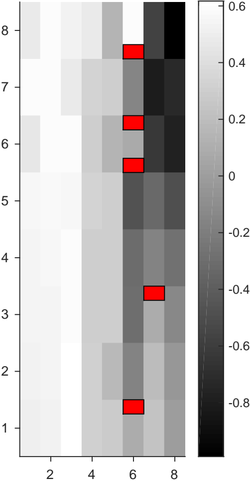
YutaMouse42-151116--DS2map _mV-trigCh7
