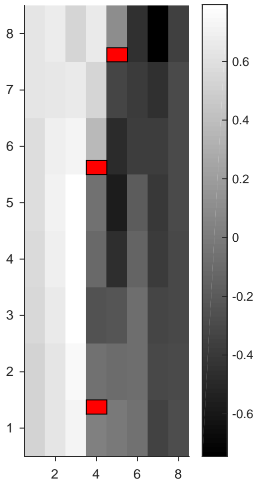
YutaMouse57-161014--DS2map _mV-trigCh26
