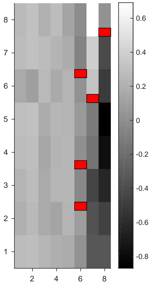
YutaMouse59-170221--DS2map _mV-trigCh48
