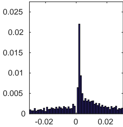
all pairID:3 preID:462 postID:472
