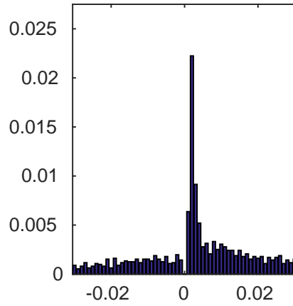
non burst spike
