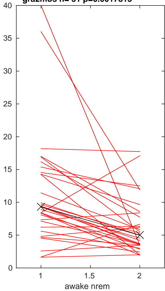
DG a5 II --SpikeTransmission--Awake-NREM--gra2mos--median gra2mos n= 31 p=0.0017813
