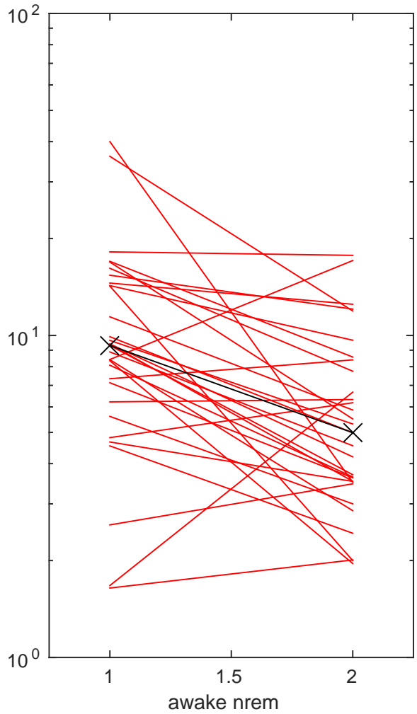
DG a5 II --SpikeTransmission--Awake-NREM--gra2mos--median gra2mos n= 31 p=0.0017813
