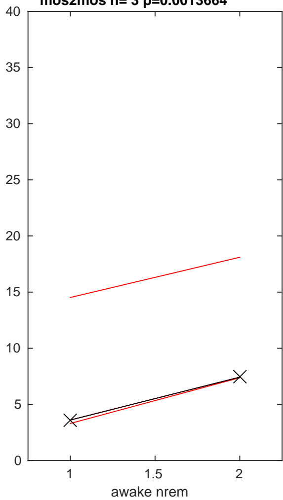
DG a5 II --SpikeTransmission--Awake-NREM--mos2mos--median mos2mos n= 3 p=0.0013664
