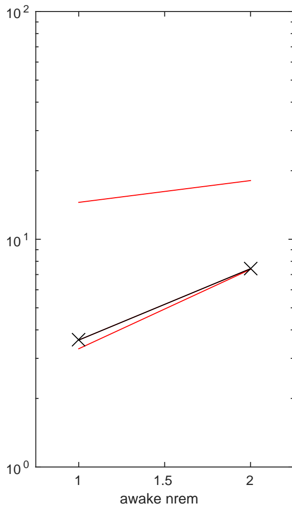
DG a5 II --SpikeTransmission--Awake-NREM--mos2mos--median mos2mos n= 3 p=0.0013664
